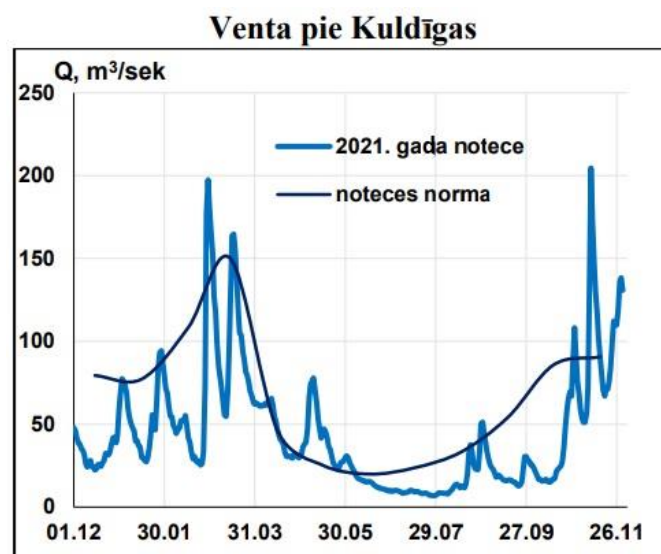
9. attēls. Ventas upes notece 2021. gadā salīdzinājumā ar ilggadīga perioda noteci (avots: LVĢMC)
